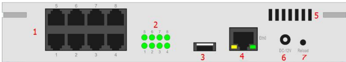
图 1-3-2 背面端口
