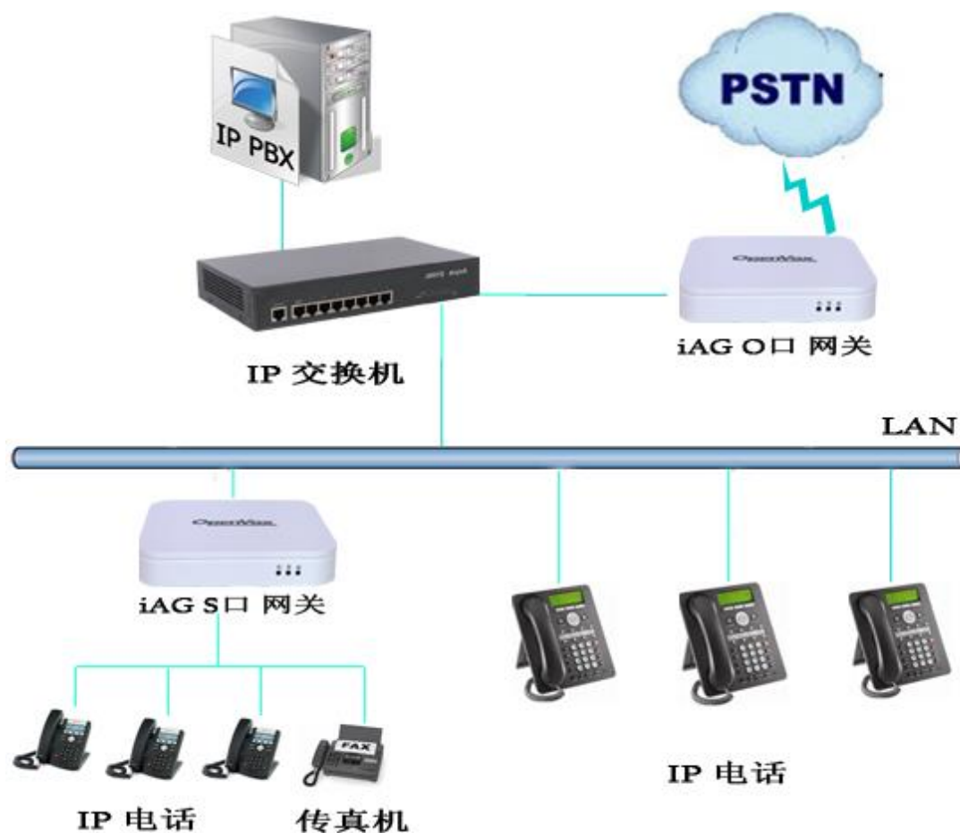
图 1-2-1 应用拓扑图
