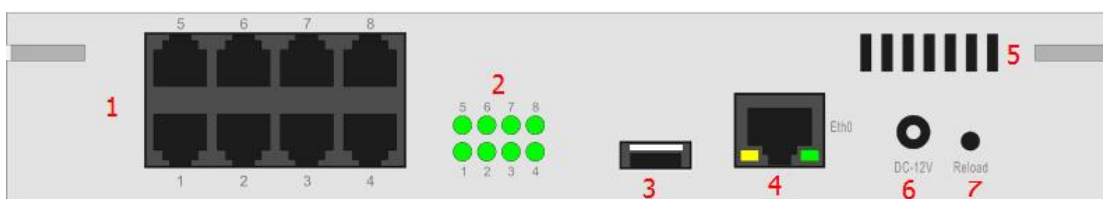
图 1-3-2 背面端口
