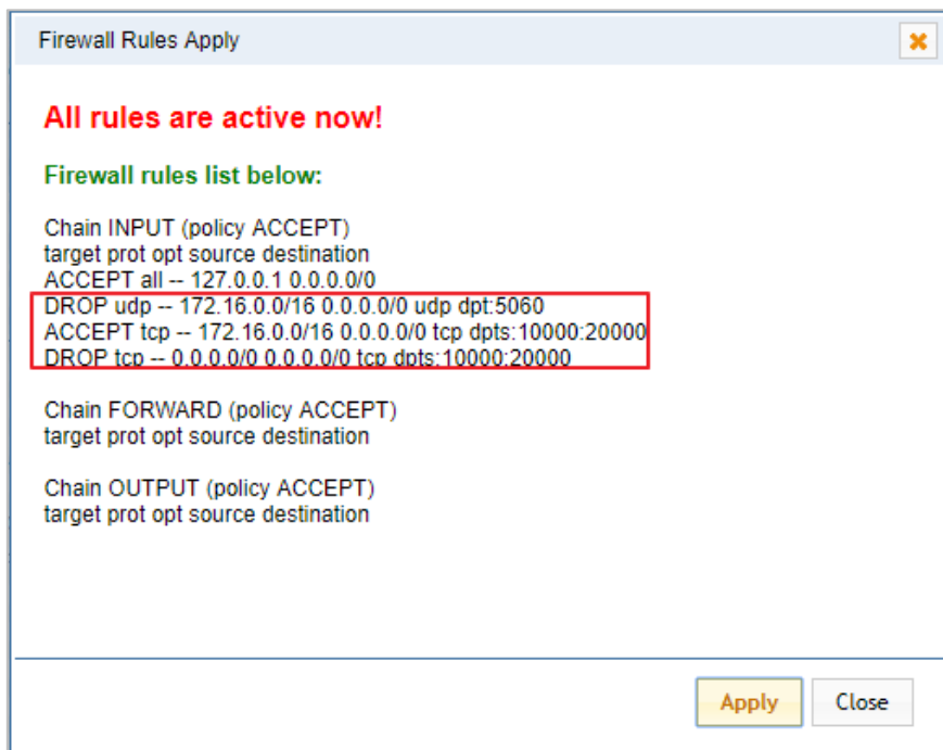
图 7-7-3 防火墙规则应用
