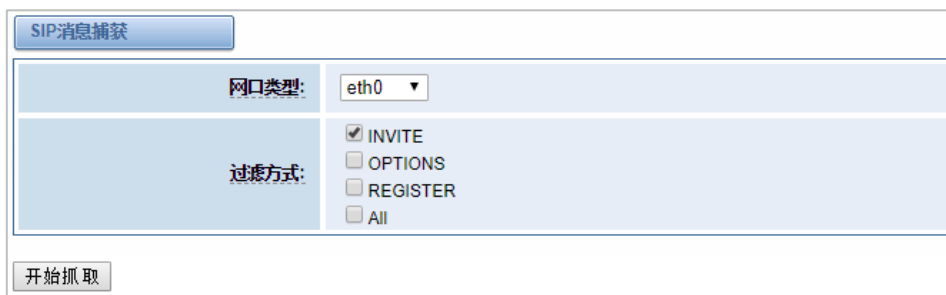
图 7-8-1 SIP 抓包
