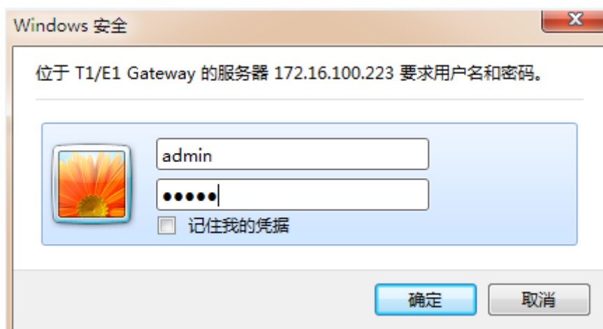
图 1-6-1 登入界面
