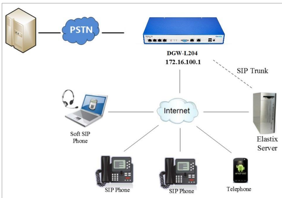
图 1-2-1 拓扑图
