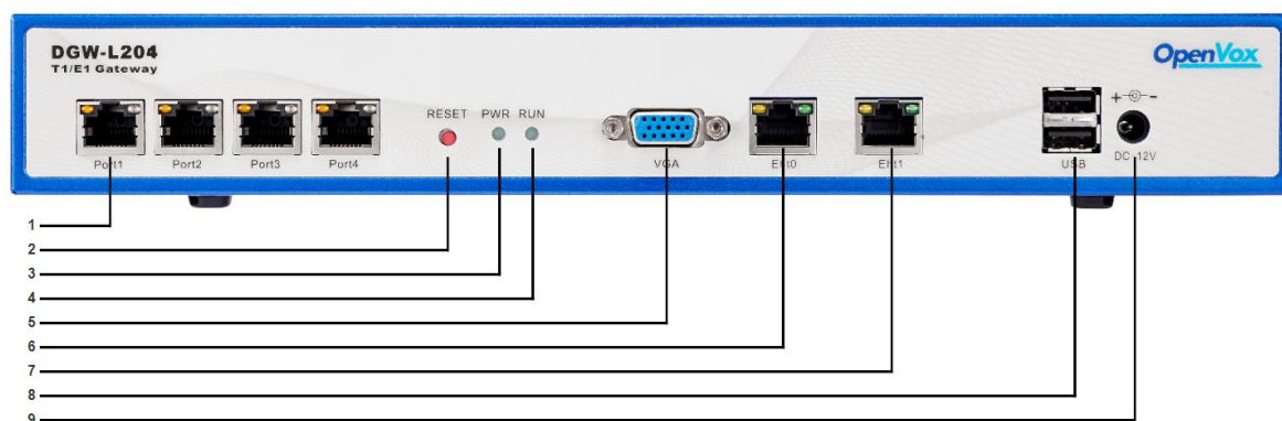
图 1-3-2 前板
