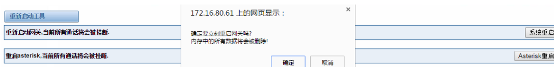
图 2-5-1 重启提示
