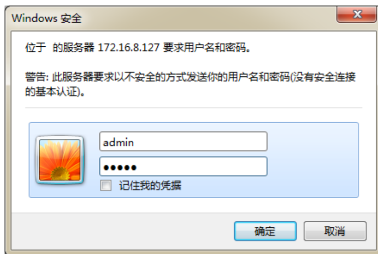
图 1-6-1 登陆界面
