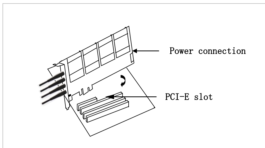
图6 硬件安装
