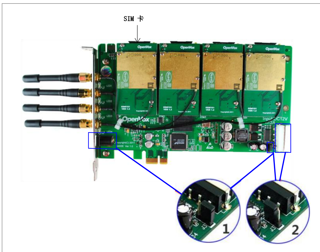
图 3 两种供电方式
